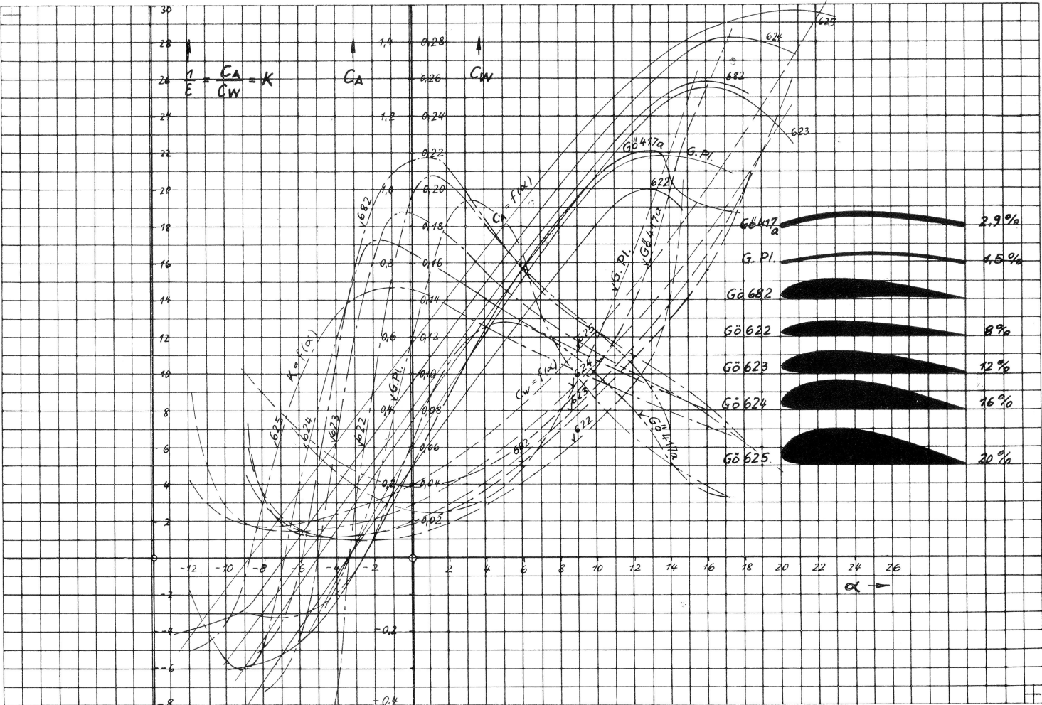
Bild 2.38 Aerodynamische Kennwerte für Luftschraubenprofile (für Flügelstreckung \lambda = 5 )
