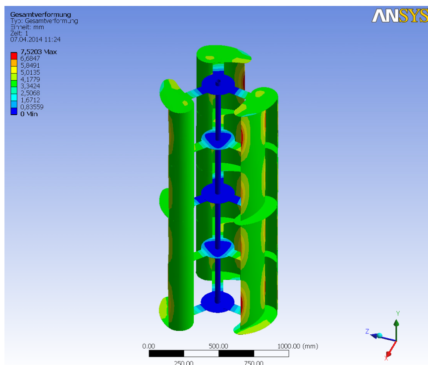
Abbildung 14 Gesamtverformung, nur durch Fliehkräfte und Gewicht
