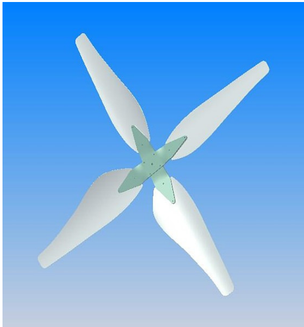
Abbildung 20 Normalwindrad Ø 1,5 m TSR 4
