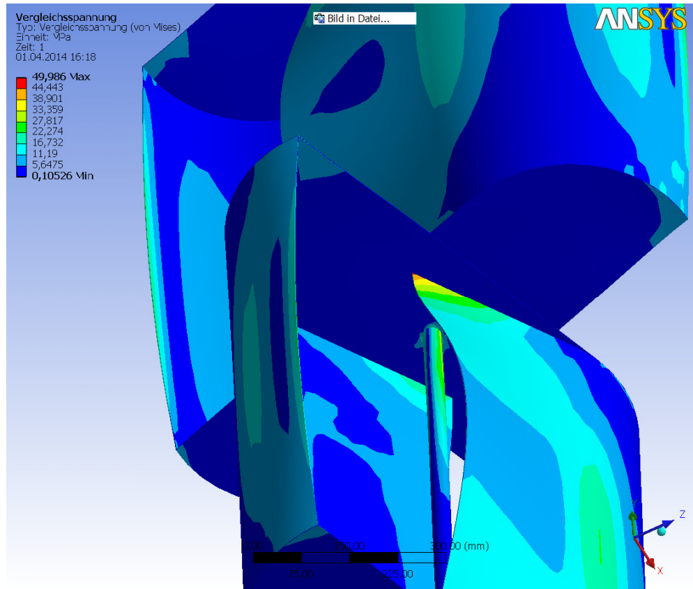
Abbildung 6 Spannungszustand, vergrößert
