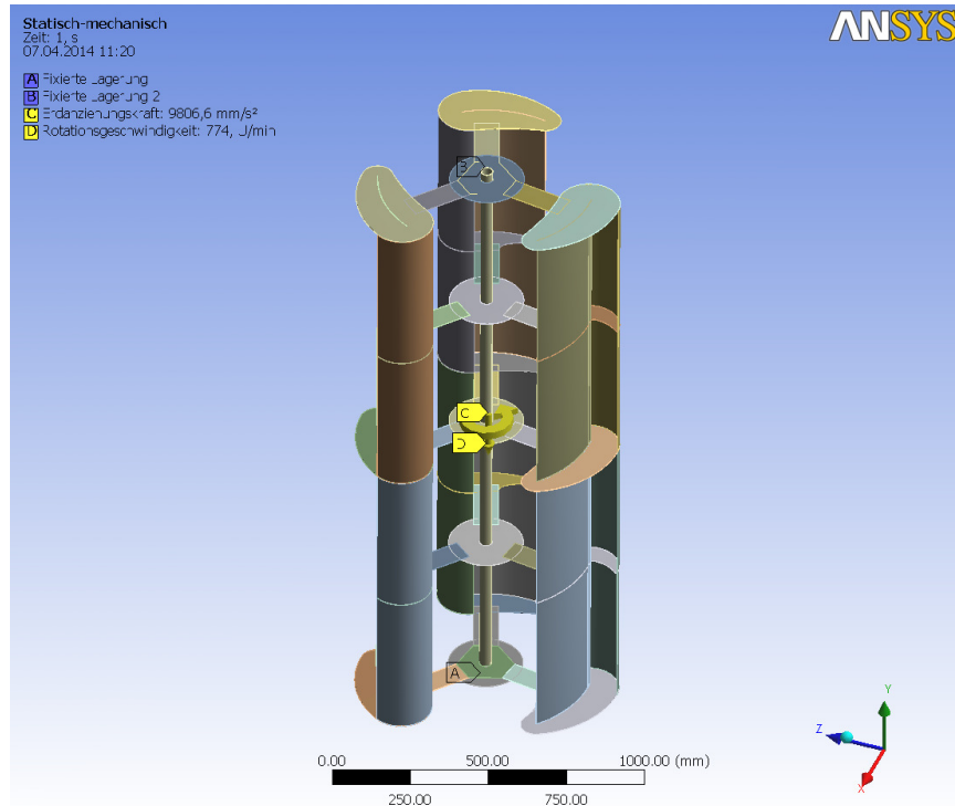
Abbildung 13 Konstruktion mit Randbedingungen, Leerlauf-TSR 1,5 (keine Luftkräfte)
