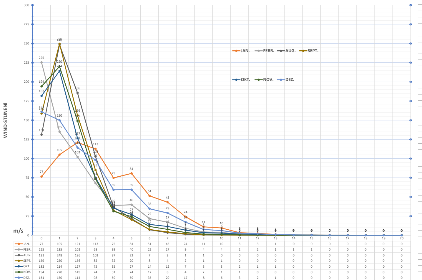
WINDSTUNDEN nach MONATEN und m/s 1.8.2018 - 28.02.2019
