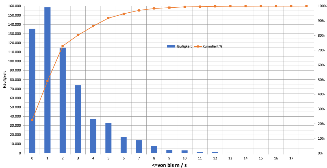
WIND - Histogramm - Häufigkeiten m / s 30-Sek.-Werte - 1.8.2018 - 28.02.2019
