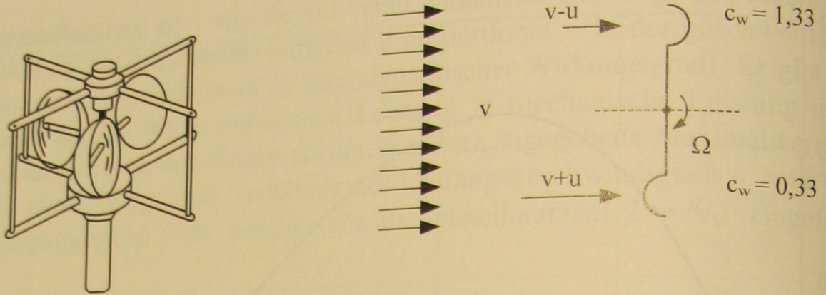
Bild 2-22 a) Schalenkreuzanemometer b) Ersatzmodell
