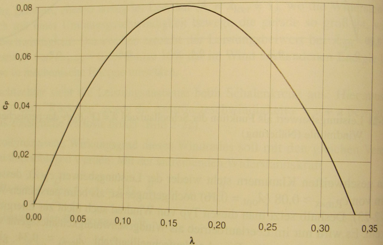
Bild 2-23 Leistungsbeiwert als Funktion der Schnelllaufzahl eines Schalenkreuzanemometers (Näherung)
