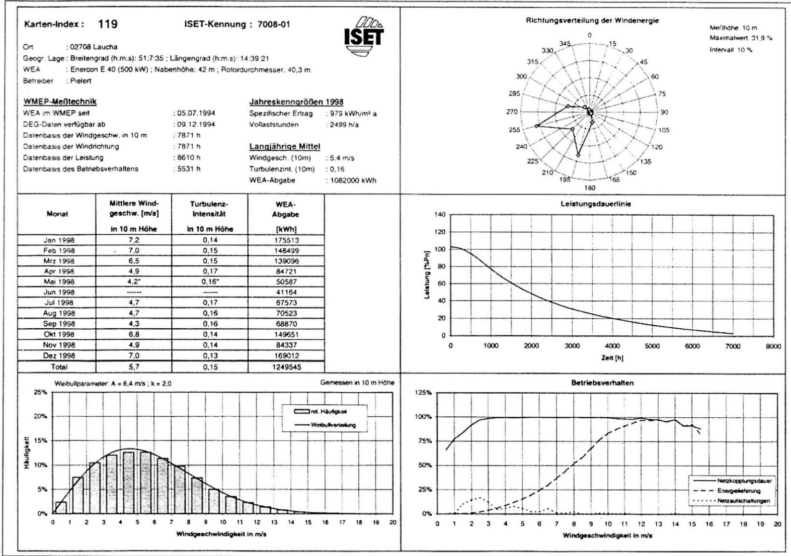
Abb. 20: Einzelergebnisse der Datenauswertung zur Standortcharakterisierung im Breitenestprogramm „250 MW Wind“ (ISET) für einen Binnenlandstandort
